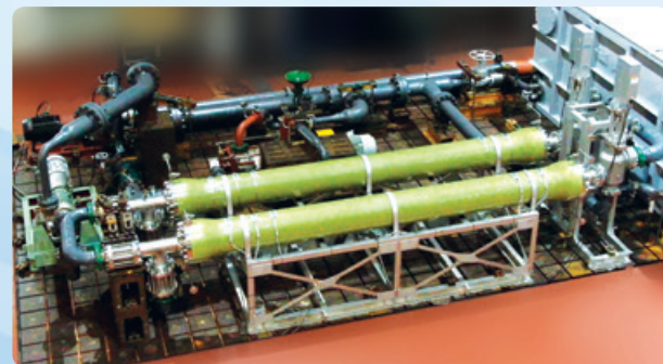
逆浸透膜法海水淡水化用エネルギー回収装置 (DeROs®)
